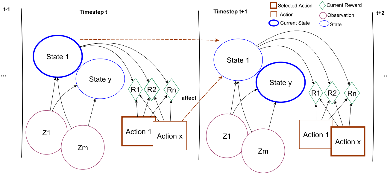
Fig. 2 MR-POMDP
