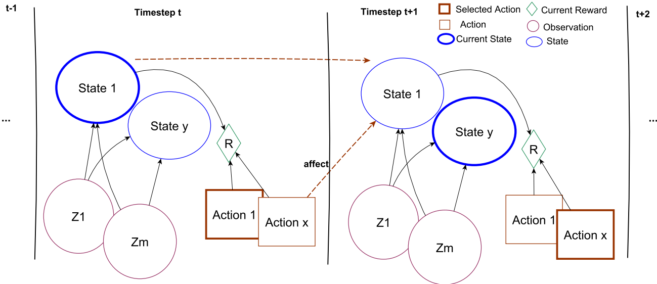
Fig. 1 POMDP
