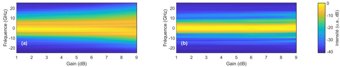
Fig. 4 : Evolution du spectre optique du signal amplifié en sortie de la fibre optique en fonction du gain de l'amplificateur Raman : (a) sans correction externe de la SPM, (b) avec modulation de phase appliquée.
